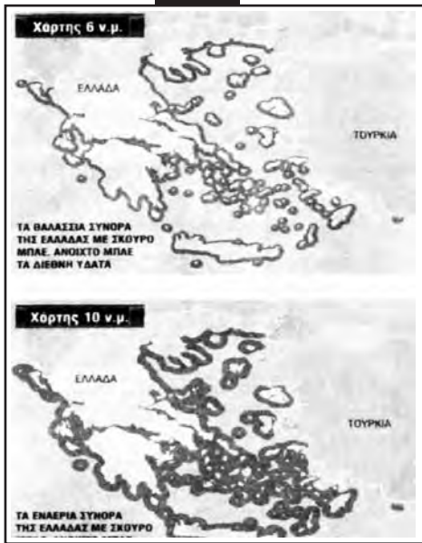
Εικόνα 1. Τα έξι και τα δέκα ναυτικά μίλια και τι σημαίνουν για το Αιγαίο. Η εικόνα και η σχετική περιγραφή από το περιοδικό Αυτό/ #10, 7/2006.
