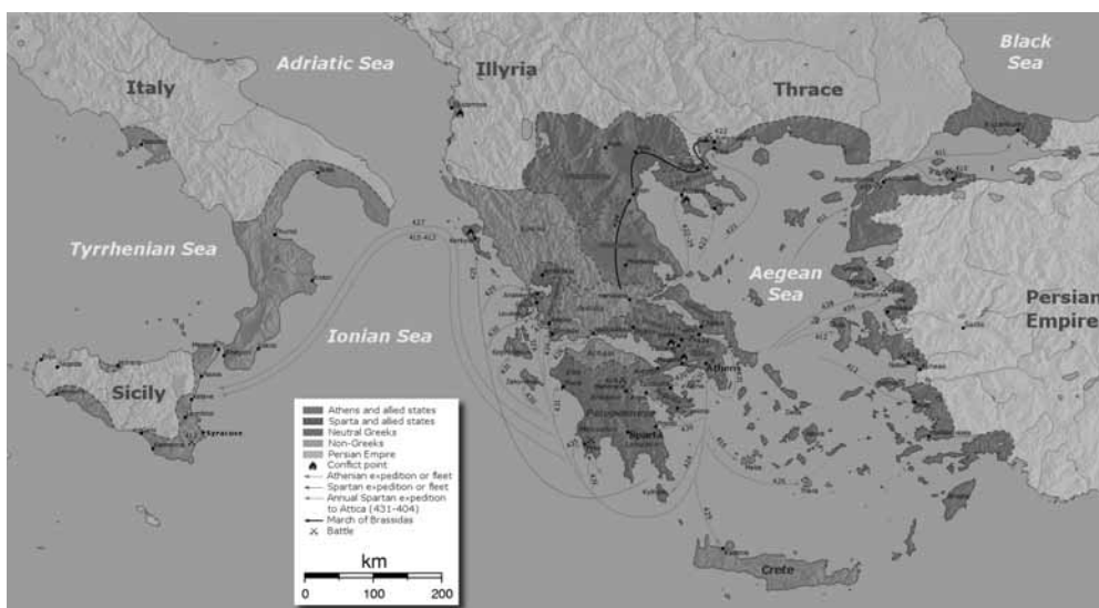
Το πεδίο στρατιωτικών επιχειρήσεων του Πελοποννησιακού Πολέμου. Προσέξτε ότι τα πλοία ήταν αναγκασμένα να κινούνται παραλιακά. Συνεπώς για να πάνε στη Σικελία, έπρεπε να περάσουν από την Κέρκυρα. Είναι αυτό που λέμε για τη «θέση» ως συνάρτηση της τεχνικής και των παραγωγικών δυνατοτήτων.
